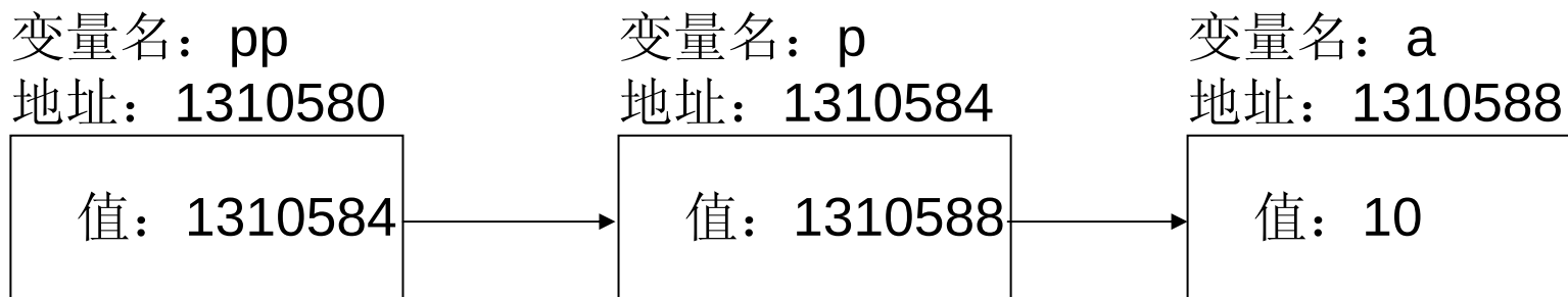
图10.1.3 多重指针关系示意图
