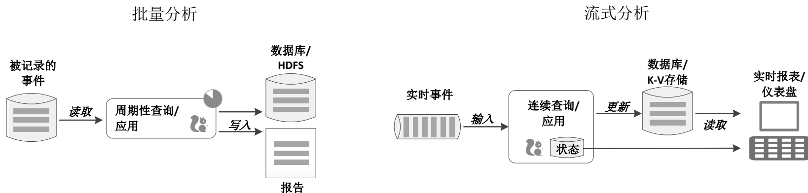
图 Flink同时支持流式及批量分析应用
