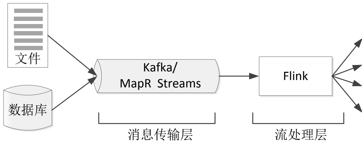
图 流处理架构
