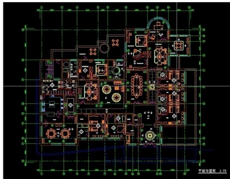
施工图
