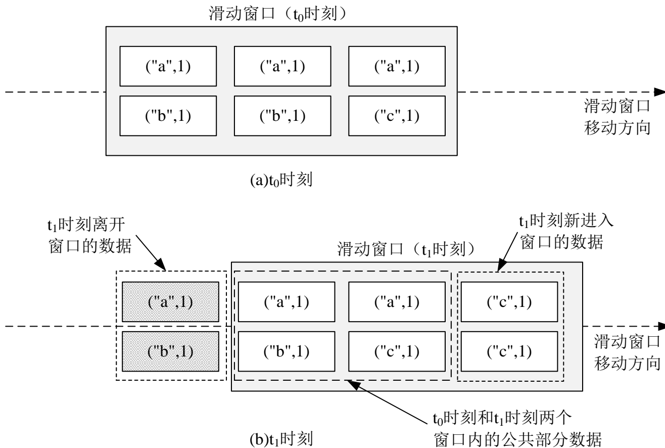
图 reduceByKeyAndWindow操作过程示意图
