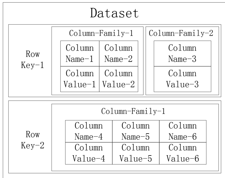
列族数据库
